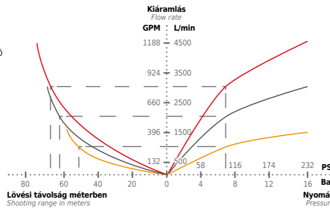
AUTOKADOR 5000 SUGÁRCSŐ DIFFUSER AUTOKADOR 5000
